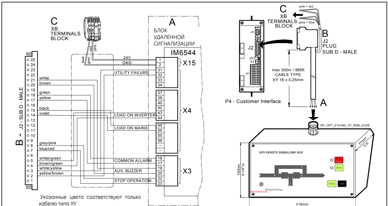
Рис. 10.5.3-1 Подключение удаленного сигнального устройства
