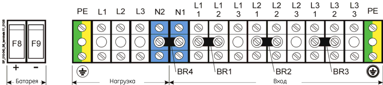
Рис. 5.8-1 Доступ к кабельным клеммам
