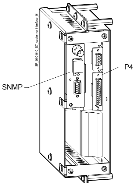
Рис. 2.1-5 Блок интерфейсов
